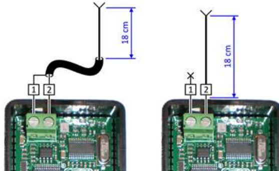
2.Ábra: antenna bekötése
