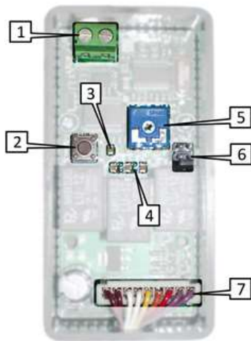
1.Ábra: a modul felépítse
